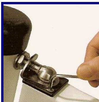
Charnières à ressort
