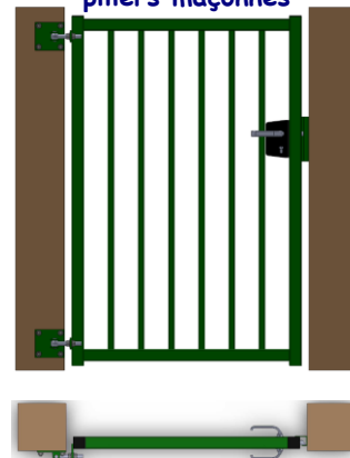
Vue intérieure fixation sur piliers maçonnés
