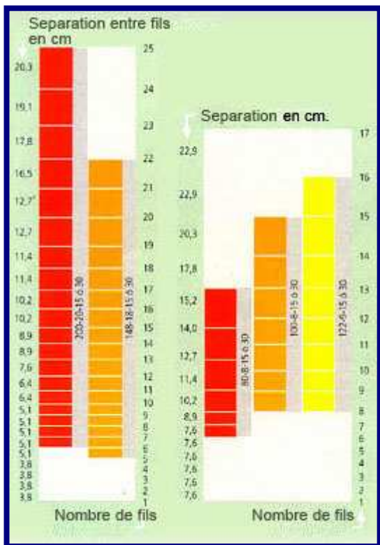
Ecart en cm entre les fils verticaux en fonction de la hauteur du rouleau.
