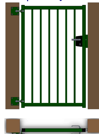
Vue intérieure fixation sur piliers maçonnés
