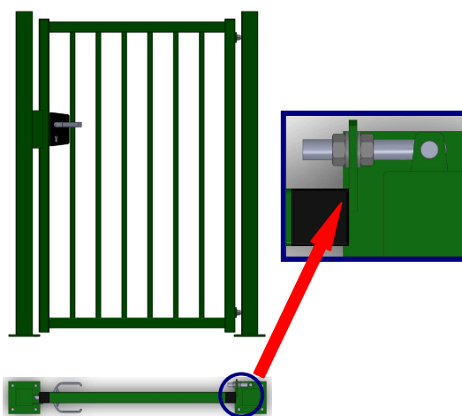
Vue intérieure piles sur platine
