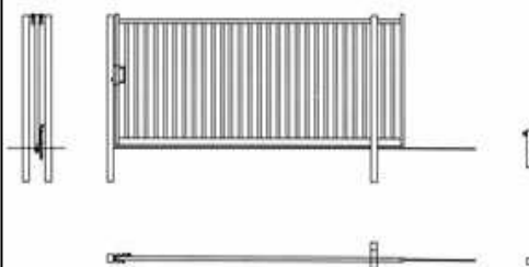
Vue de dessus du portail coulissant
